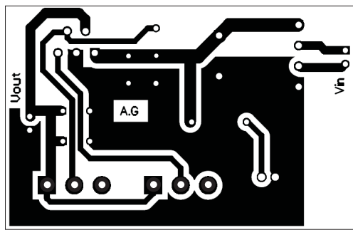
PCB - Actual size / Copper side view
